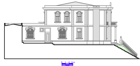
Elevação 02
