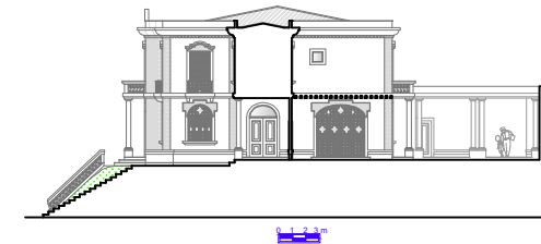
Elevação 04
